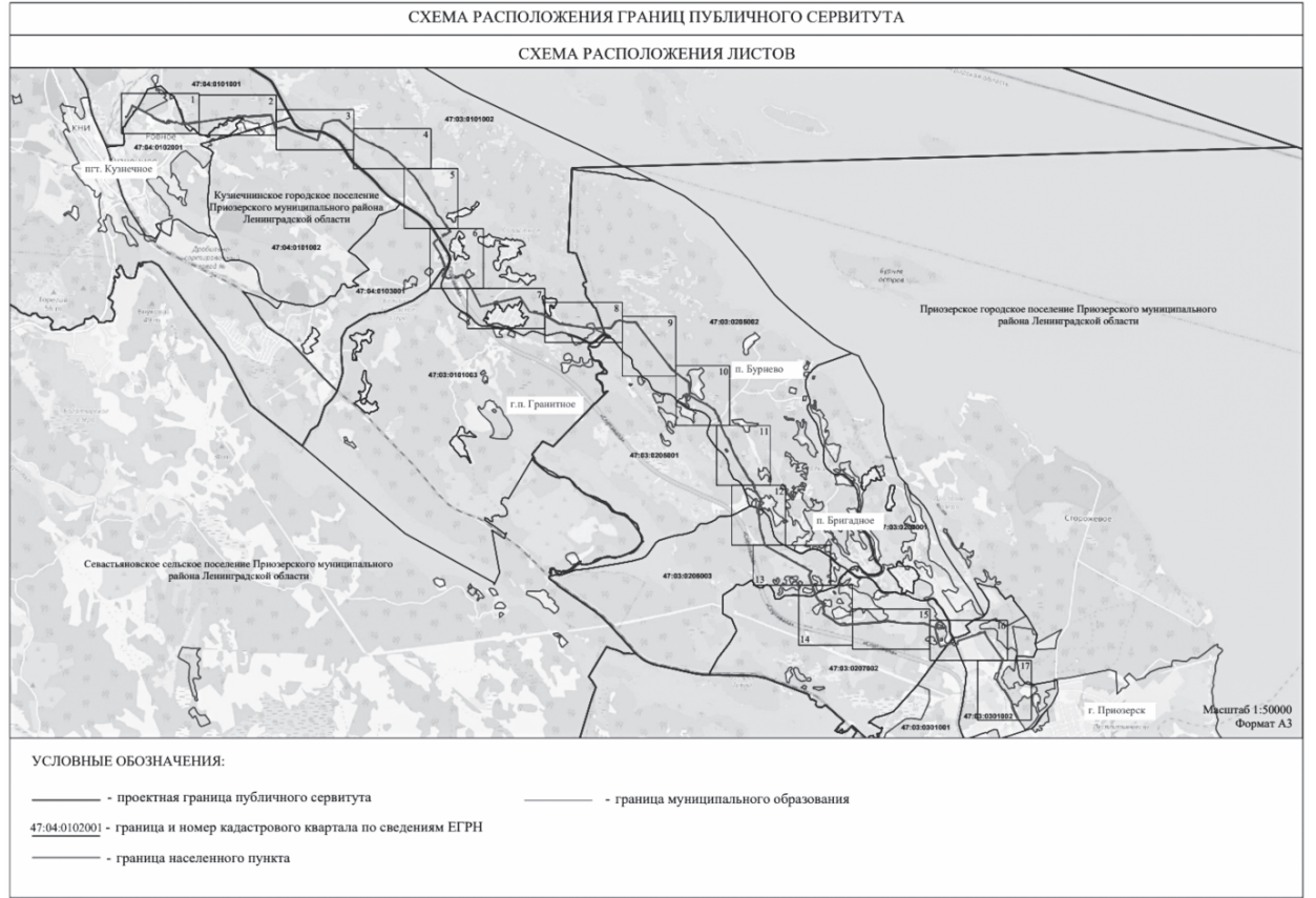
Схема расположения грани публичного сервитута "Распределительный газопровод по пос. Суходолье" Приложение к ходатайству об установлении публичного сервитута
